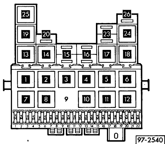
Relaisplatzbelegung
